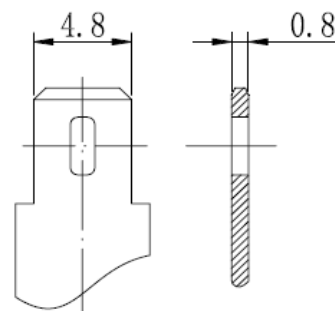
Позиция клемм
